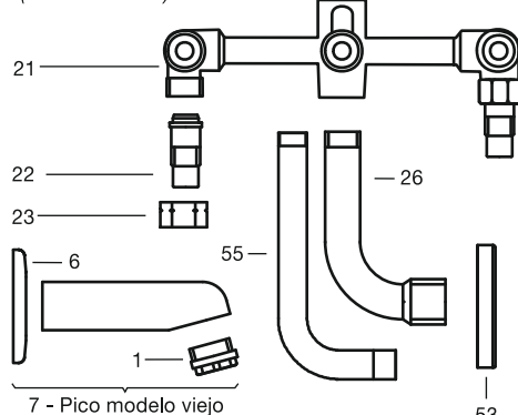
Esqueleto para juego 0109 (anterior a 2007)
