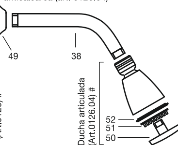
Ducha articulada completa anticalcárea (art. 0120,04)
