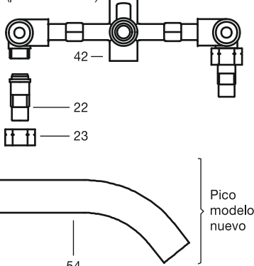
Esqueleto para juego 0109 (posterior a 2007)
