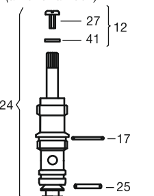
Cabeza transferencia (anterior a 2007)
