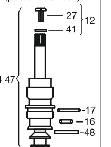
Cabeza transferencia (posterior a 2007)
