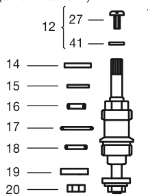
Cabeza (anterior a 2007)
