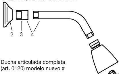
Ducha articulada completa (art. 0120) modelo hasta 2002 #
