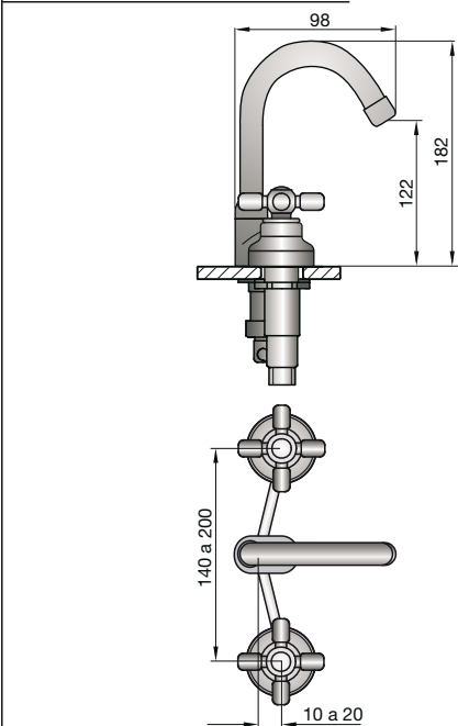
Art. 0212 (Lavatorio con tapita)
