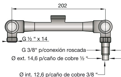
Esqueleto del juego 109 (para ducha)
