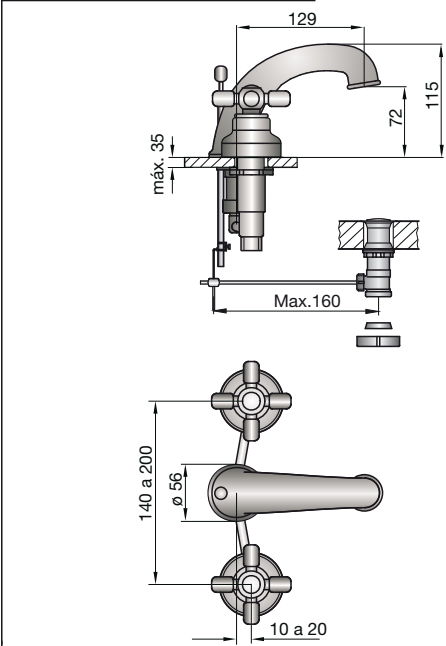
Art. 0201 (Lavatorio a pistón) Art. 0207 (Lavatorio con tapita)
