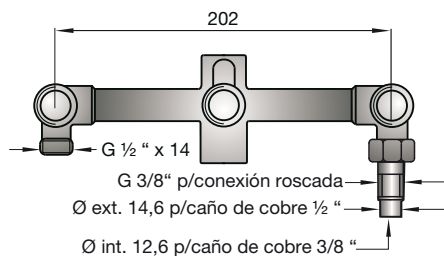
Esqueleto del juego 109 (para ducha)
